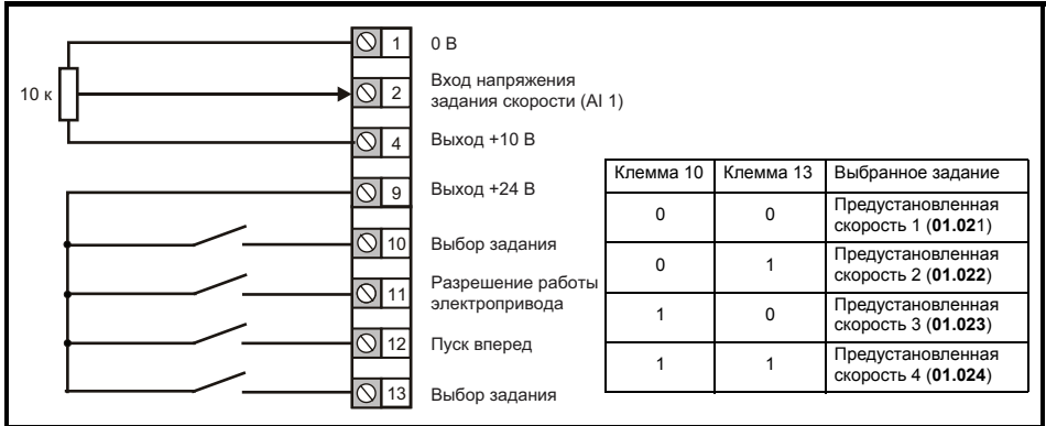
Рис. 4-9 Pr 00.005 = Preset (50 Гц)
