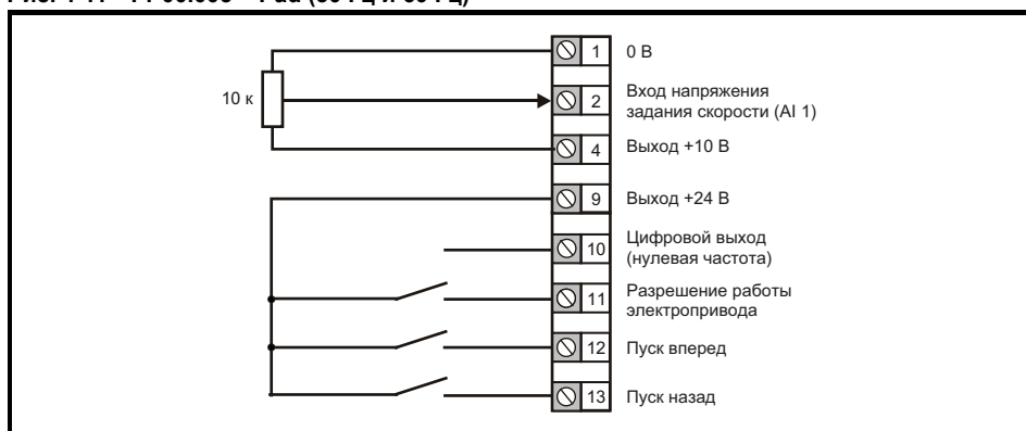
Рис. 4-11 Pr 00.005 = Pad (50 Гц и 60 Гц)
