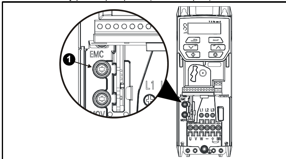
Рис. 4-15 Снятие внутреннего фильтра ЭМС (показан габарит 2)
