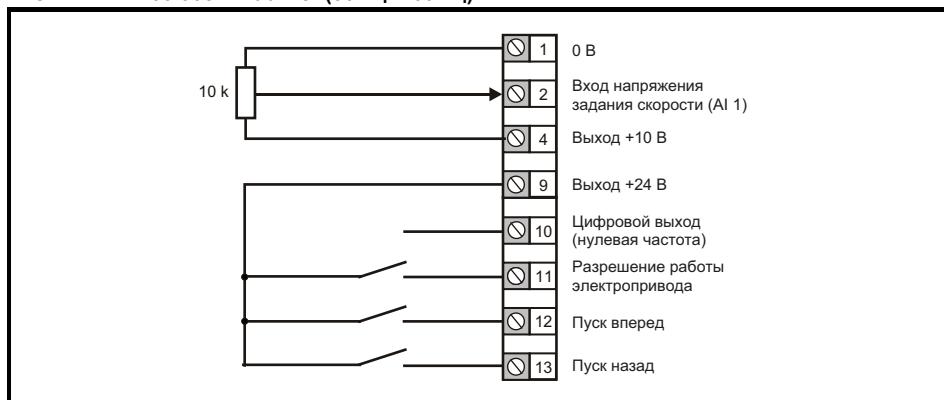
Рис. 4-12 Pr 00.005 = Pad.Ref (50 Гц и 60 Гц)
