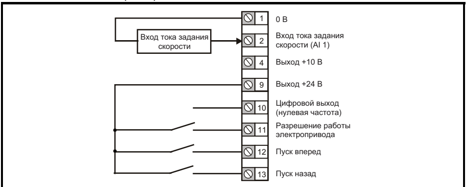
Рис. 4-3 Pr 00.005 = AI (50 Гц)
