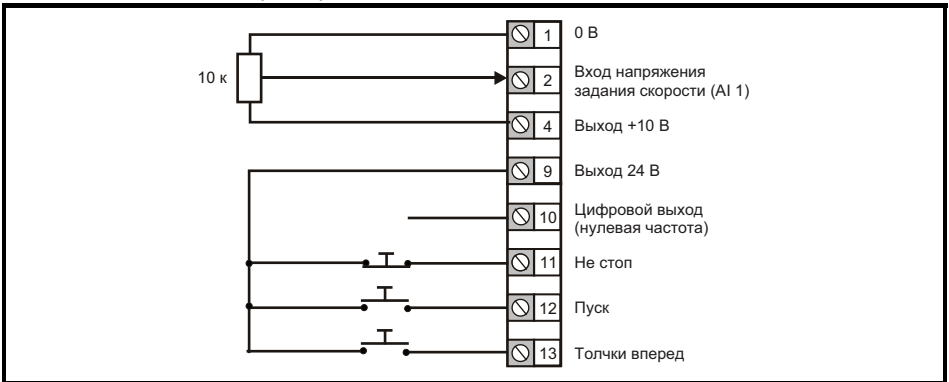
Рис. 4-2 Pr 00.005 = AV (60 Гц)
