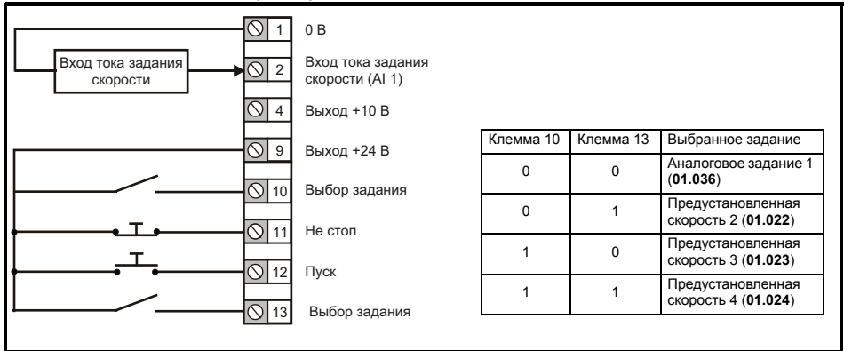
Рис. 4-8 Pr 00.005 = AV.Pr (60 Гц)
