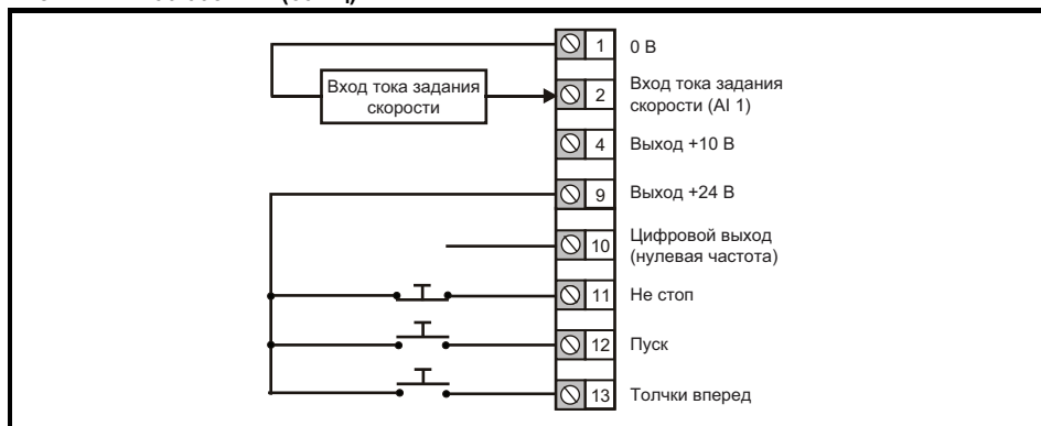
Рис. 4-4 Pr 00.005 = AI (60 Гц)
