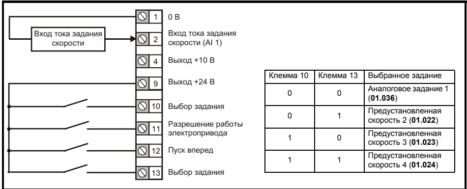
Рис. 4-7 Pr 00.005 = AV.Pr (50 Гц)
